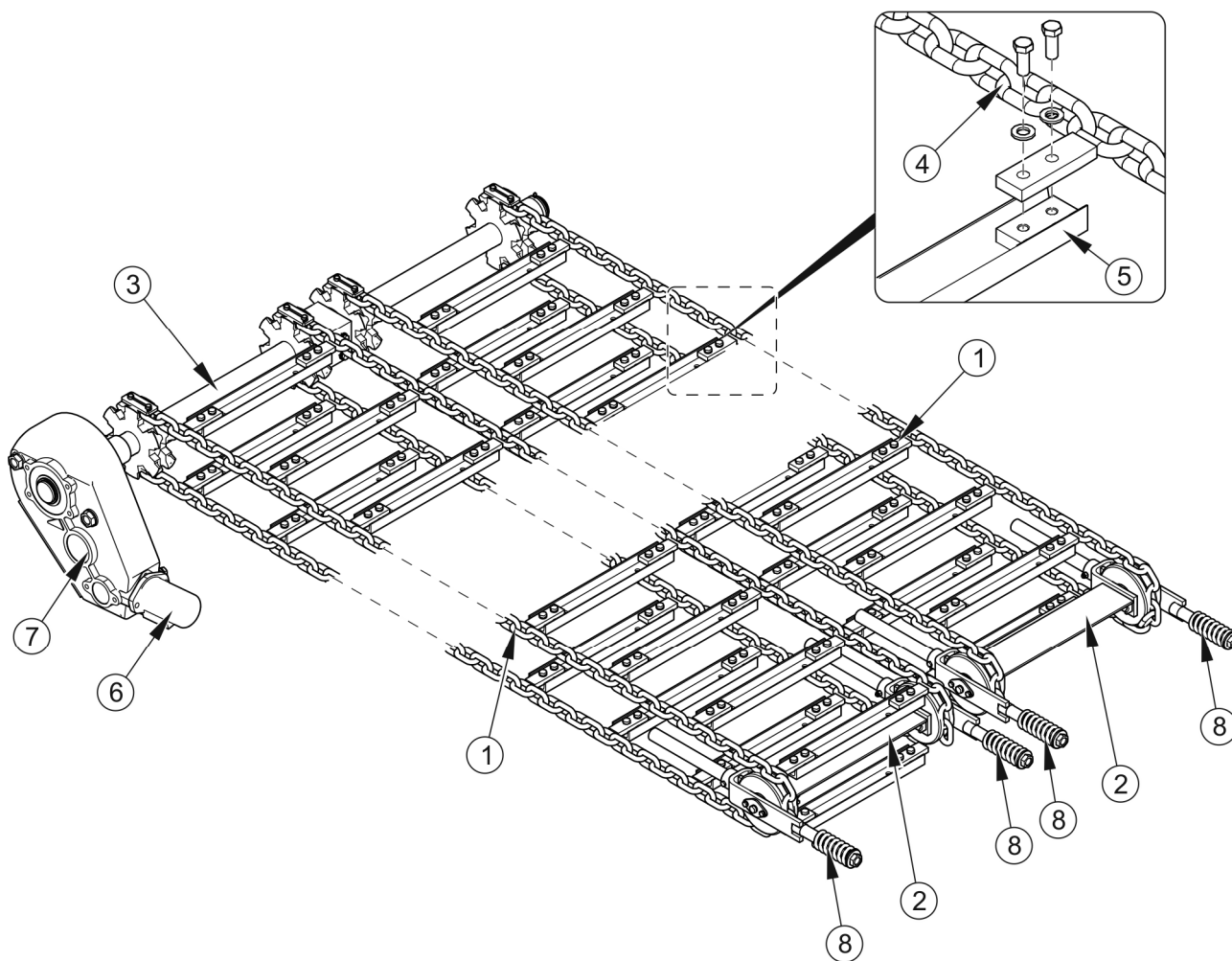
RYSUNEK 3.3 Mechanizm podający NV161/4, NV161/5
