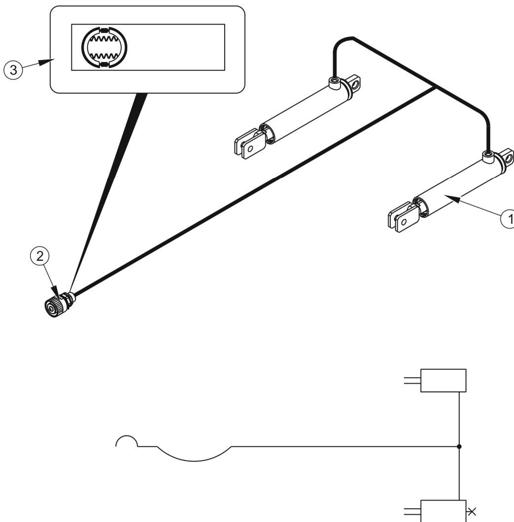
RYSUNEK 3.11 Budowa i schemat instalacji hamulcowej hydraulicznej
