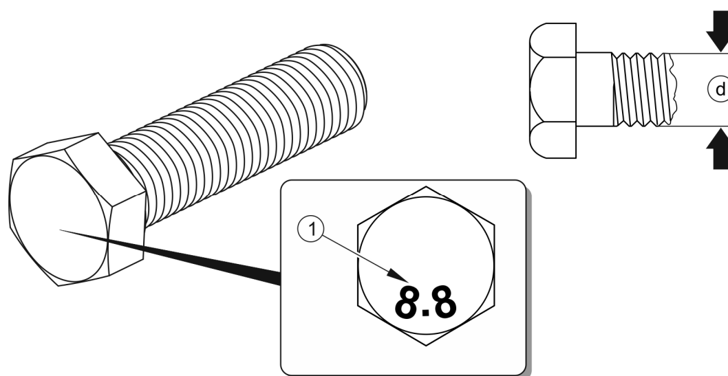
RYСУNEK 5.17 Śruba z gwintem metrycznym
