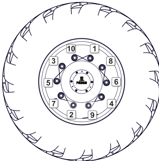
RYSUNEK 5.4 Kolejność dokręcania nakrętek, osie z 10 szpilek M22x1.5
