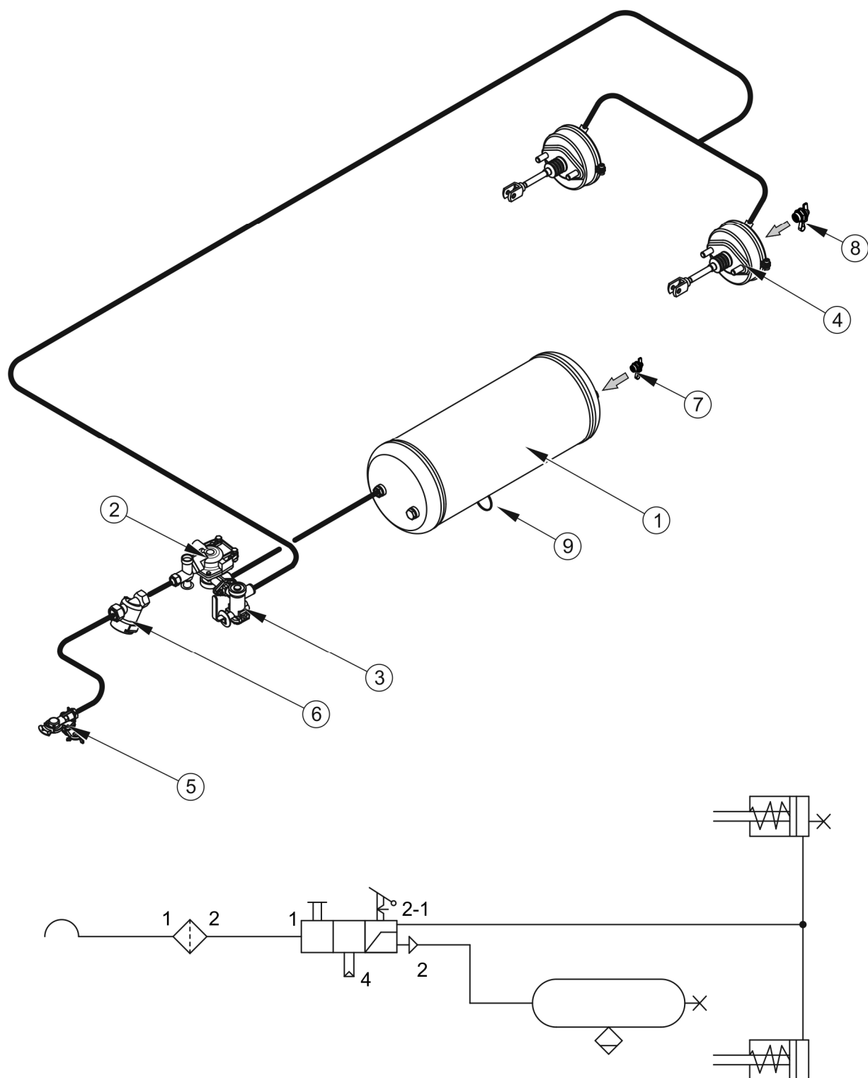
RYSUNEK 3.9 Instalacja pneumatyczna jedнопроводова
