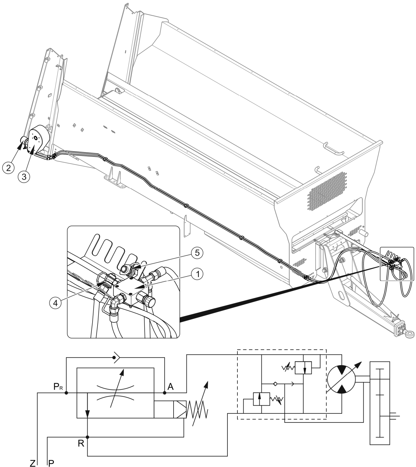
RYSUNEK 3.4 Budowa i schemat instalacji hydraulicznej mechanizmu podającego
