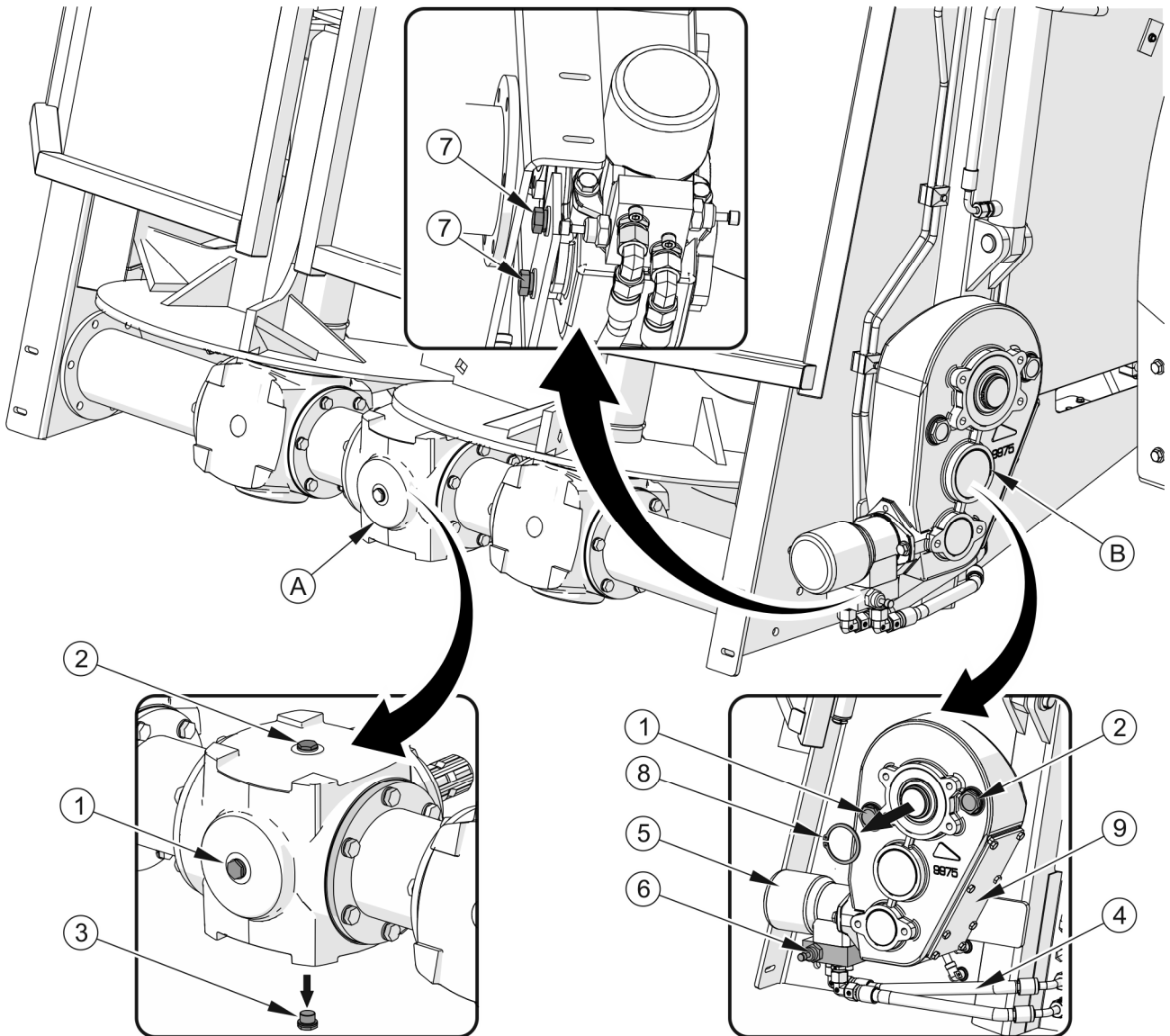
RYСУNEK 5.12 Kontrola i wymiana oleju przekładni rozrzutnika
