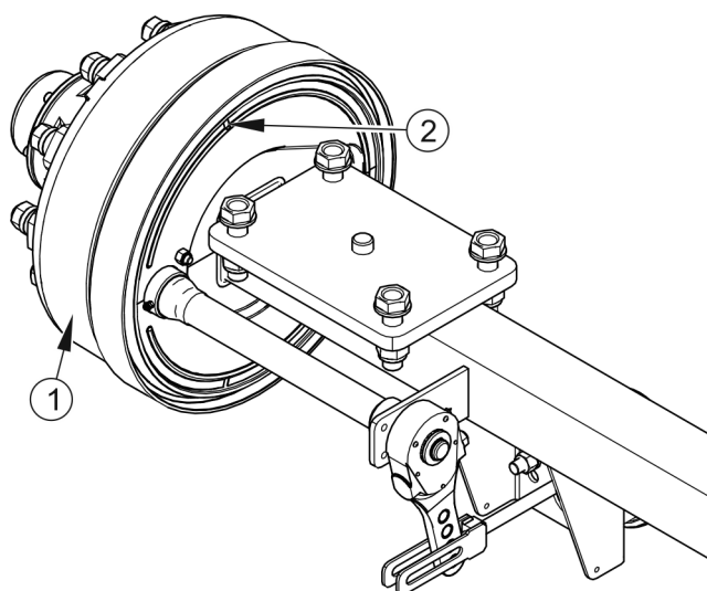
RYSUNEK 5.1 Kontrola okładzin hamulcowych
