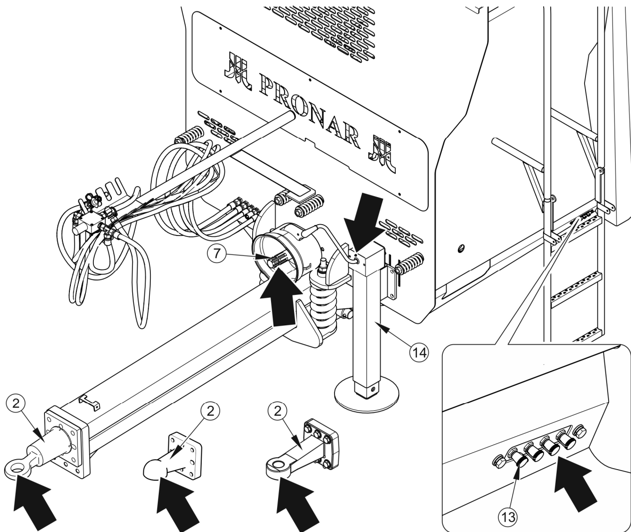
RYСУNEK 5.13 Punkty smarne rozrzutnika
